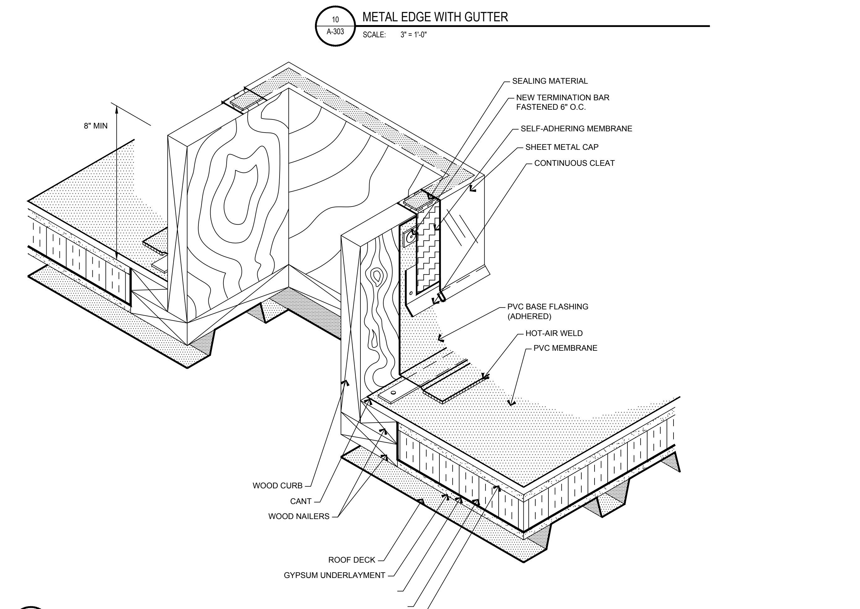
12 CURBED PENETRATION A-303 SCALE: 3" = 1'-0"
