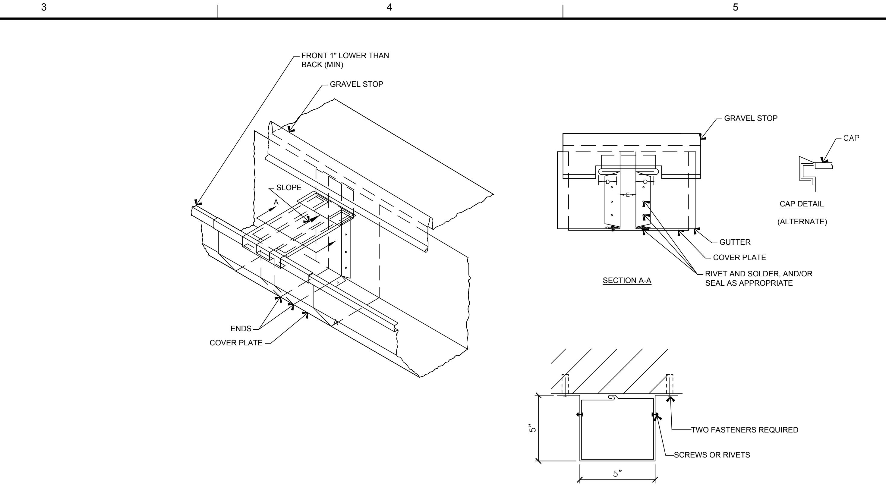
10 METAL EDGE WITH GUTTER A-303 SCALE: 3" = 1'-0"
