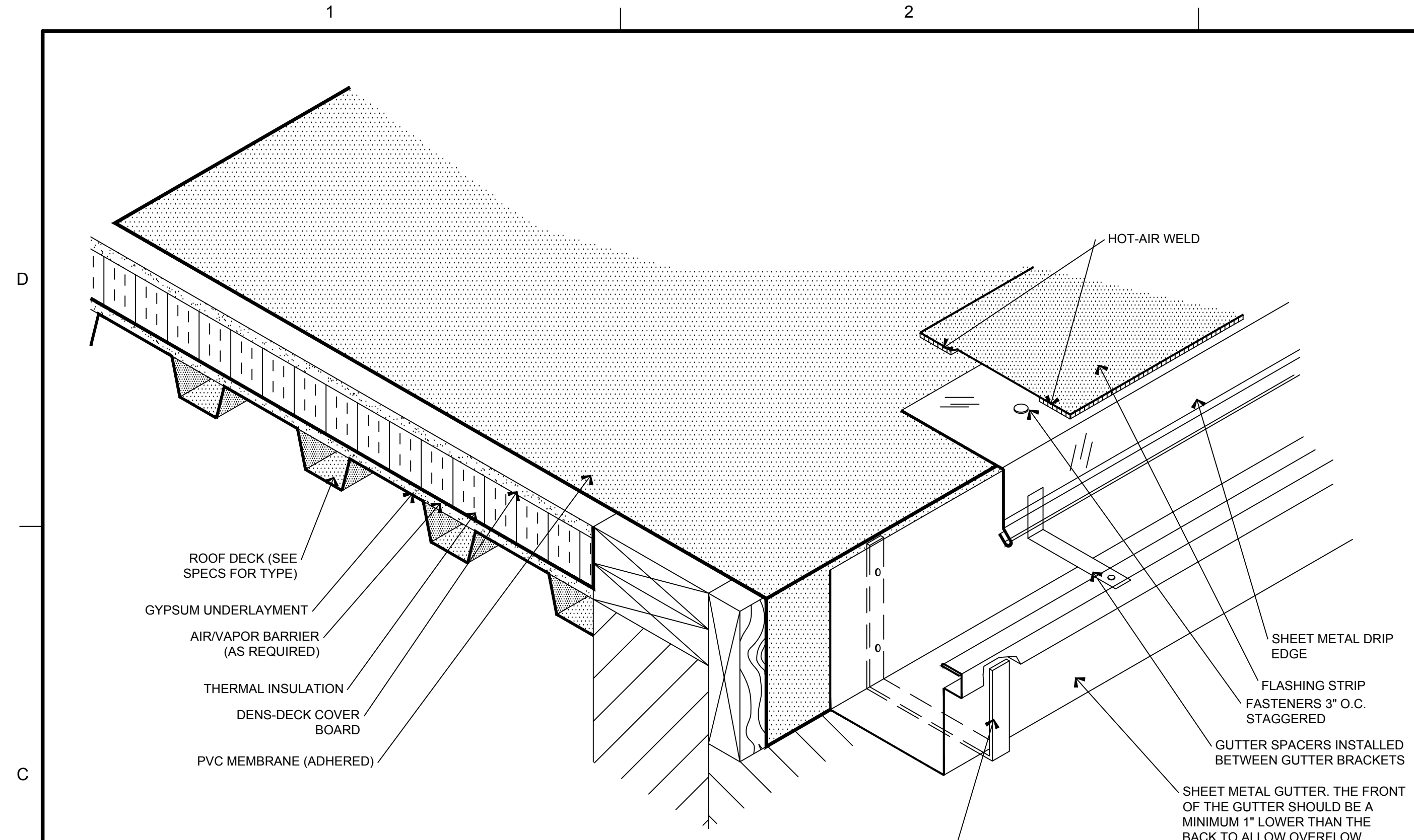
09 DRIP EDGE WITH GUTTER A-303 SCALE: 3" = 1'-0"
